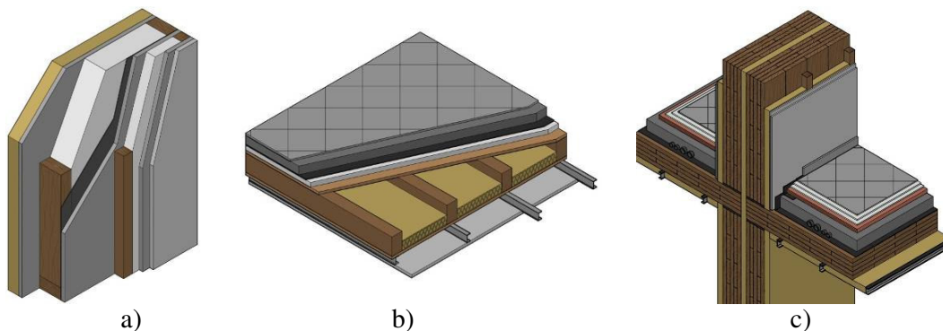
Figura 6 – dettagli costruttivi: a) parete intelaiata, b) solaio telaio, c) divisoria x-Lam
